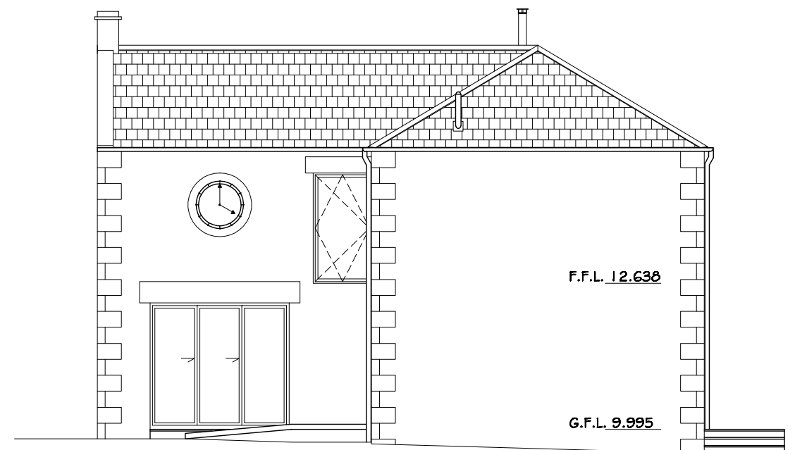
S.W. ELEVATION 1/100
