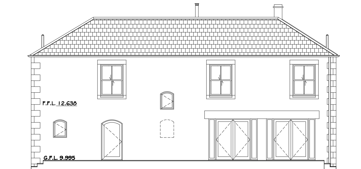
S.E. ELEVATION 1/100
