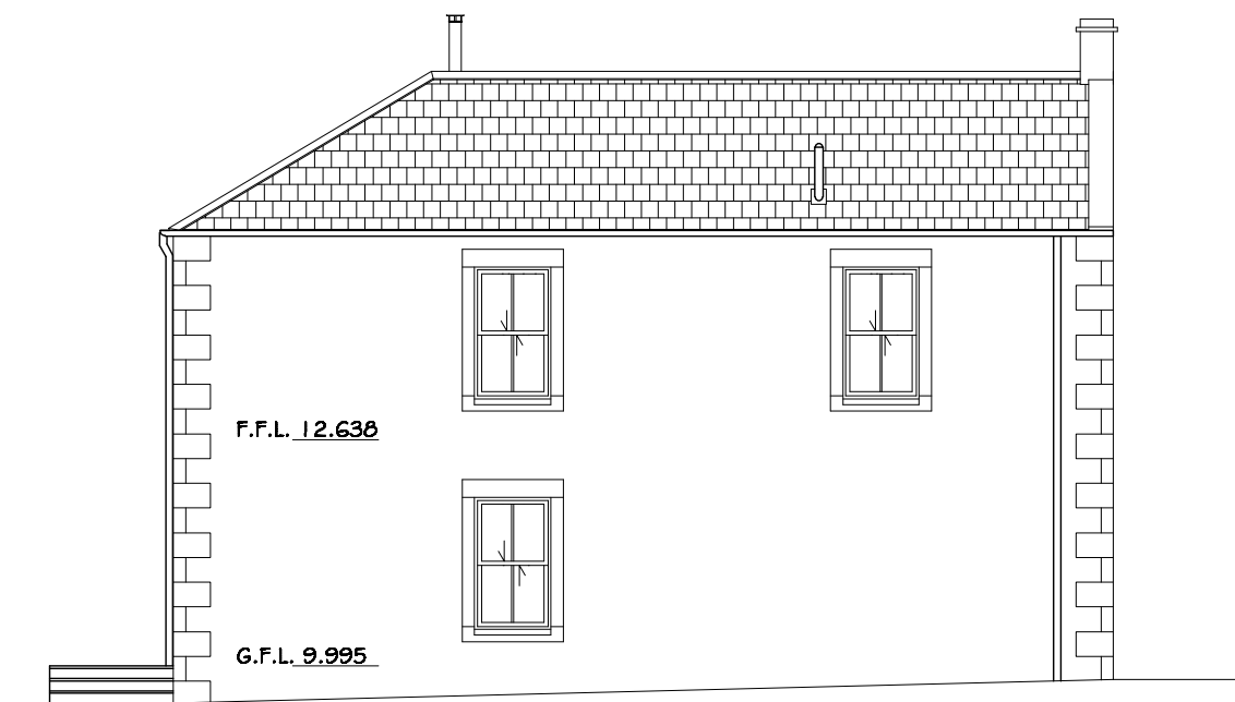
N.E. ELEVATION 1/100
